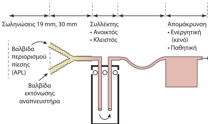
Εικόνα 14.4. Σύστημα απομάκρυνσης ή απαγωγής άχρηστων αερίων.
