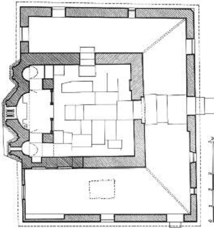
Εικ. 2. Κάτοψη του ναού των Αγίων Κηρύκου και Ιουλλίτης. Υπάρχουσα κατάσταση. Αποτύπωση 1959 (Ν.Κ.Μ.).
