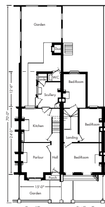
Εικ. 25. Κατοικία στο Σάφτσομπουρν Παρκ. Κάτοψη ισογείου και ορόφου (διαστάσεις οικοπέδου 4,57 επί 21,32 μ., εμβαδόν 97,43 τ.μ., εμβαδόν κατοικίας και στους δύο ορόφους 90 τ.μ.).
