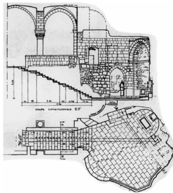
Εικ. 13. Παρεκκλήσιο της Εύρεσης. Κάτοψη-τομή (από Corbo, V.).
