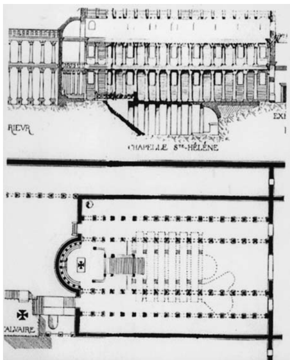
Εικ. 17. Κάτοψη και τομή-πρόταση αναπαράστασης της Βασιλικής και του υπογείου παρεκκλησίου (από Vincent, H.-Abel, F.-M.).
