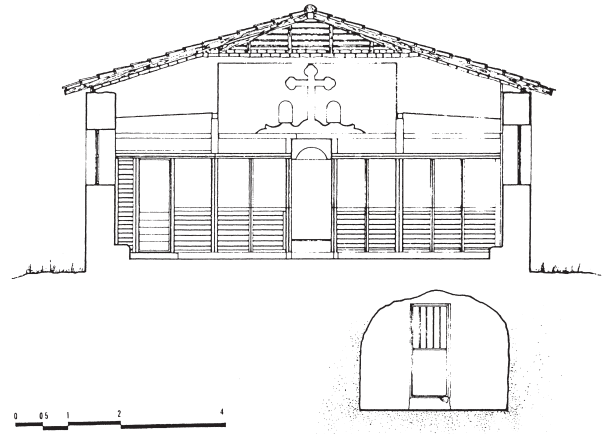
Εικ. 77. Κιβωτός. Άγιος Δημήτριος. Εγκάρσια τομή με θέα προς το Ιερό.
