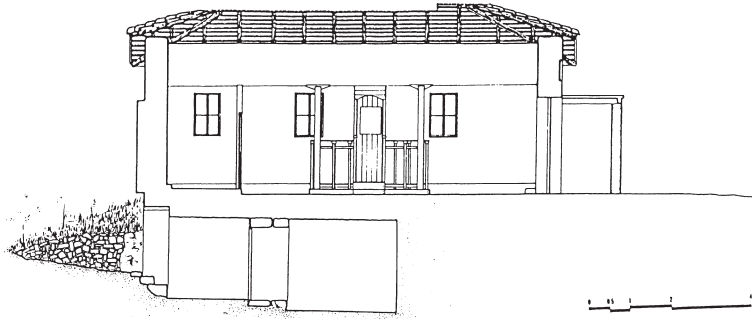
Εικ. 76. Κιβωτός. Άγιος Δημήτριος. Τομή κατά μήκος.
