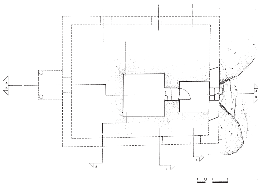
Εικ. 75. Κιβωτός Άγιος Δημήτριος. Κάτοψη υπογείου (τάφου).
