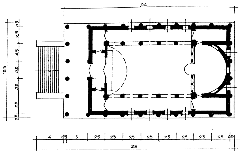
Εικ. 6. Ευαγγελισμός της Θεοτόκου Βουκουρεστίων. Κάτοψη. Fig. 6. Buna Vestire din București. Secțiune orizontală.
