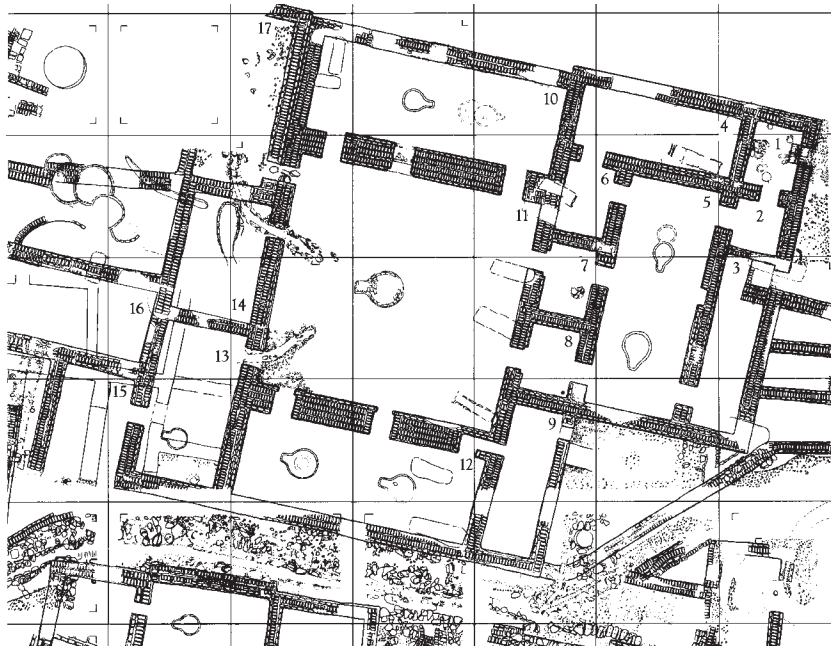
Χαμπούμπα Καμπίρα. Νοτιοανατολικό σπίτι.
