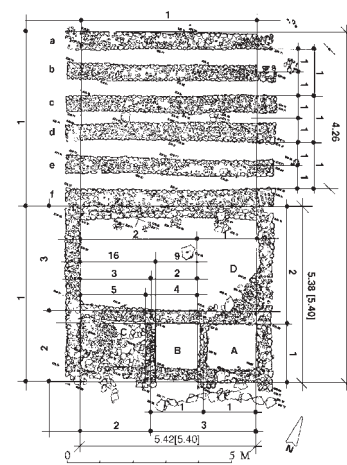
Ζαγϋϋ. Κάτοψη του στρώματος 3 με αναλογίες.
