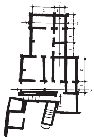
Τελ ες Σουβάν. Φάση 3Α. Σχέδια των κτισμάτων 10 και 13 με αναλογίες.
