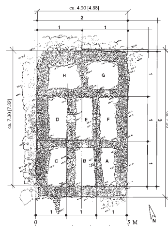
Ζαγϋϋ. Κάτοψη του στρώματος 2 με αναλογίες.
