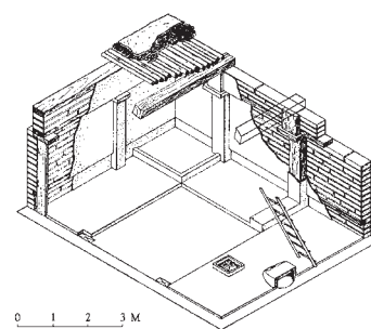
Τσατάλ Χουγιούκ. Αποκατάσταση ενός τοπικού κόριου χώρου με ανοιχτή εστία, φούρνο και σκάλα.
